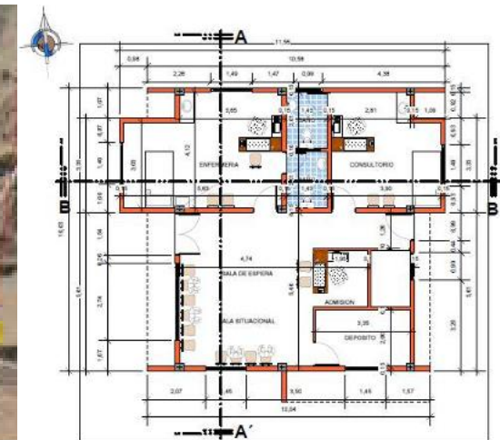
1 CORTE A-A' Escala: 1:100
