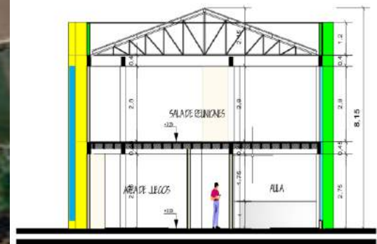
..CORTE B - B'.. ESCALA 1:100
