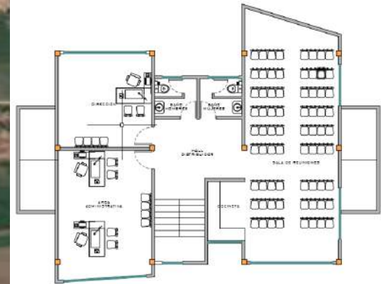
....PLANTA ALTA....
