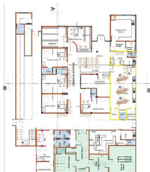
PLANO ARQUITECTONICO
